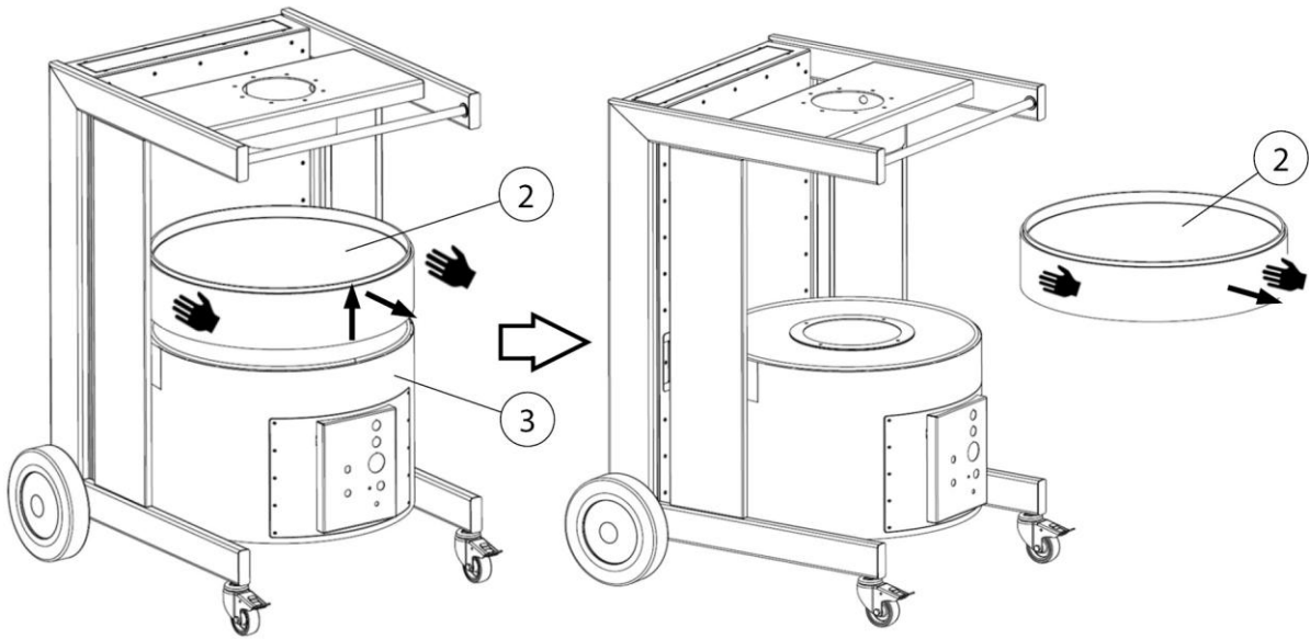
Fig 10: Cambio del filtro - extraer el filtro de carbón activo
