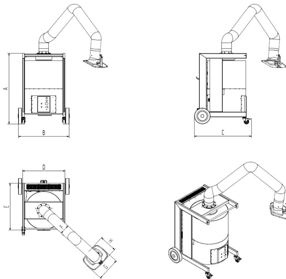
Fig. 15: Hoja de medidas
