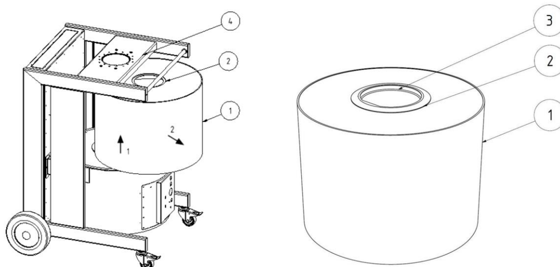
Fig. 5: Cambio de filtros
