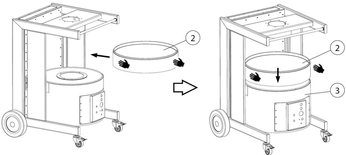
Fig 11: Cambio del filtro - Insertar el filtro de carbón activo
