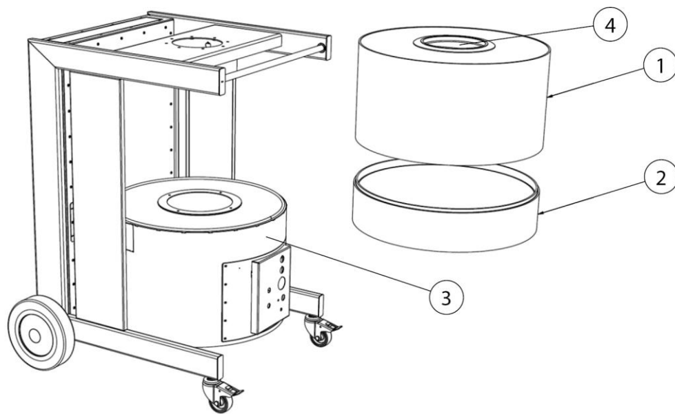
Fig 8: Sustitución del filtro
