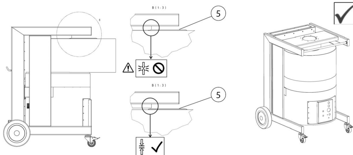
Fig 14: Cambio de filtro - comprobar junta
