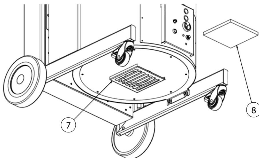
Fig. 7: Cambio del filtro de aspiración - aire de refrigeración
