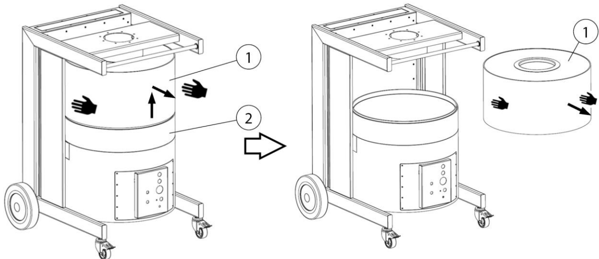
Fig 9: Cambio del filtro - Extraer el elemento filtrante
