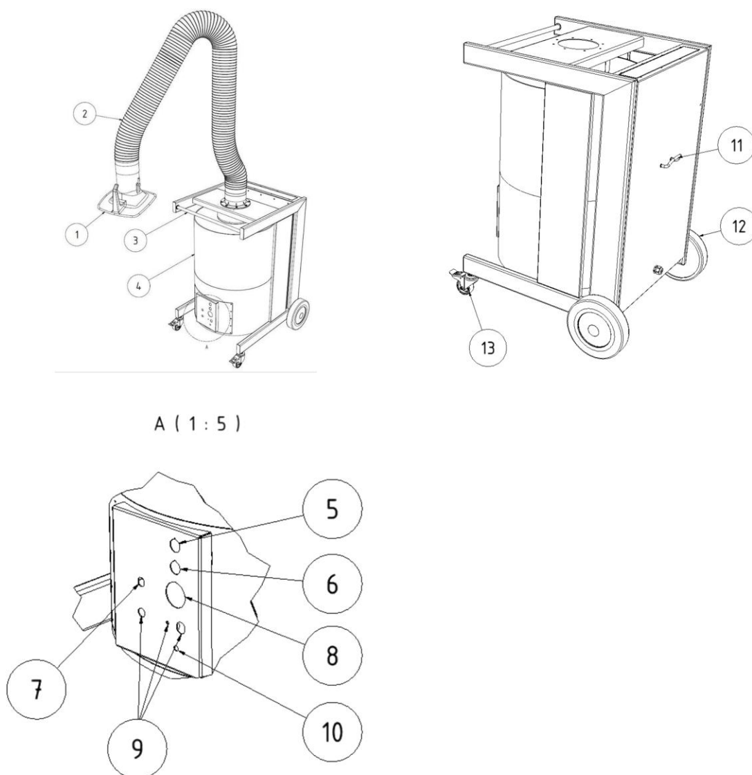
Fig. 1: Descripción del producto
